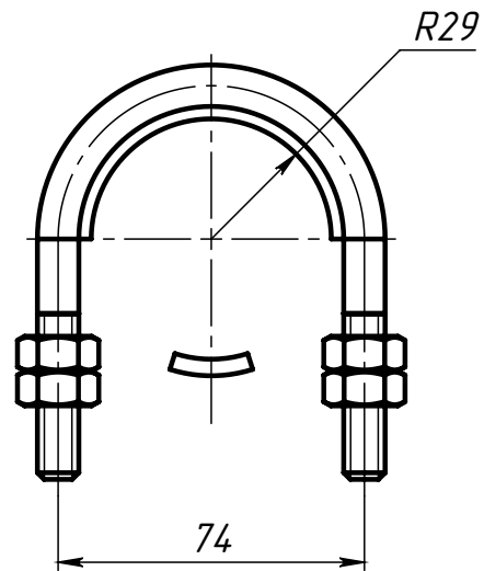
Поз.1 (Хомут)
