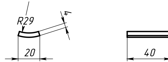
Поз.2 (Упор)
